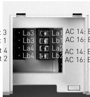
Abb. 6: Geöffnetes Anschlussfeld
