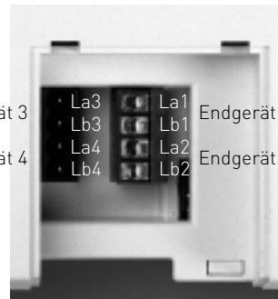
Abb. 6: Geöffnetes Anschlussfeld
